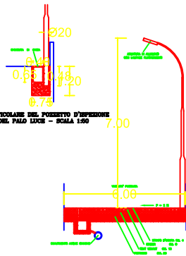
SEZIONE TIPO STRADALE - SCALA 1:50
